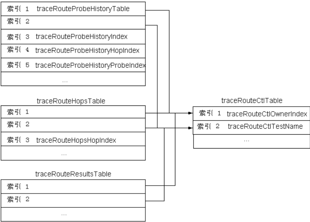
图 7-1 测试信息表与操作结果统计表的关系图
